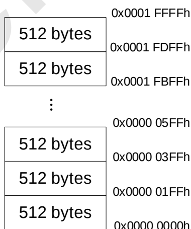
SCD515X 系列 128 Kbytes APROM Sector 分区示意
