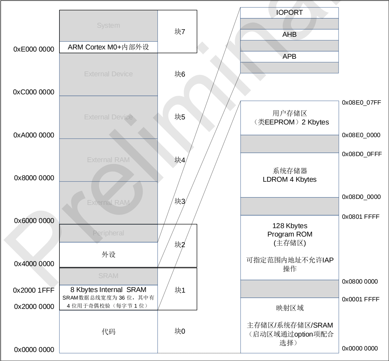
SCD515X 存储器映射图
