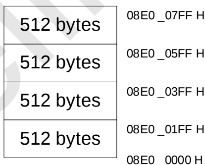
SCD515X EEPROM Sector 分区示意
