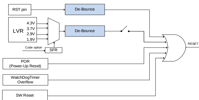
SCD515X 复位电路图
