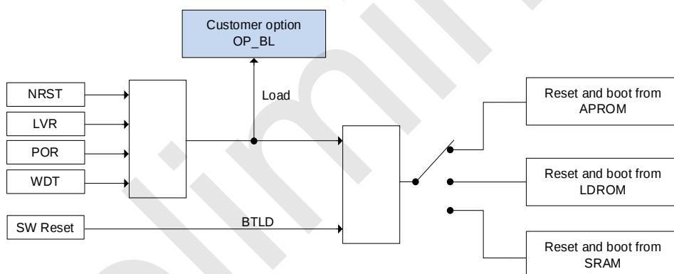
SCD515X 复位后启动区域切换示意图
