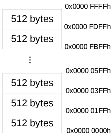
SCD515X 系列 64 Kbytes APROM Sector 分区示意
